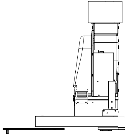
Seitenriss links
