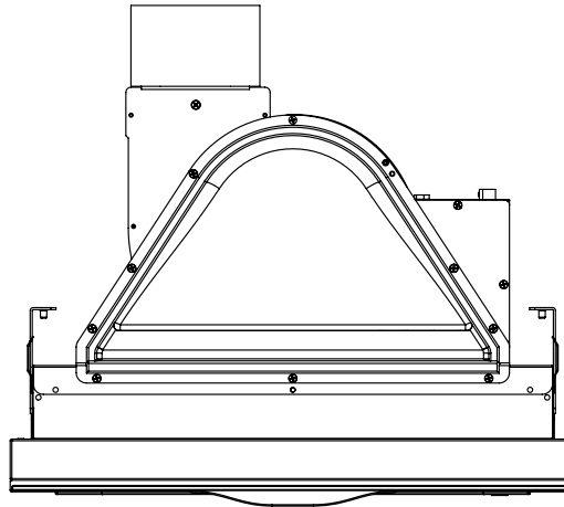
Aufriss
