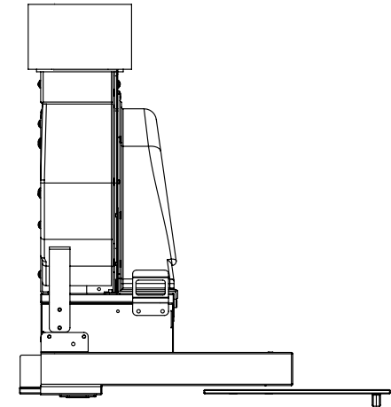
Seitenriss rechts
